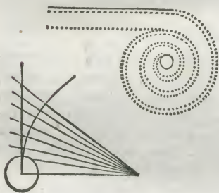
Ionicæ volutæ emendata circinatio.
